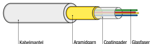
Aufbau FTTH Inhouse-Kabel 2.2mm
